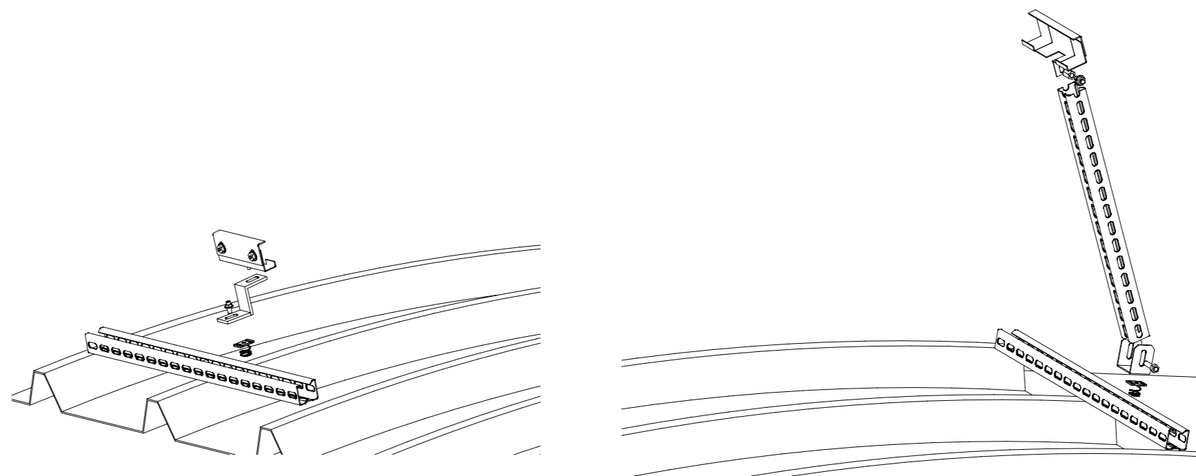
Prospetto - scala 1:10
