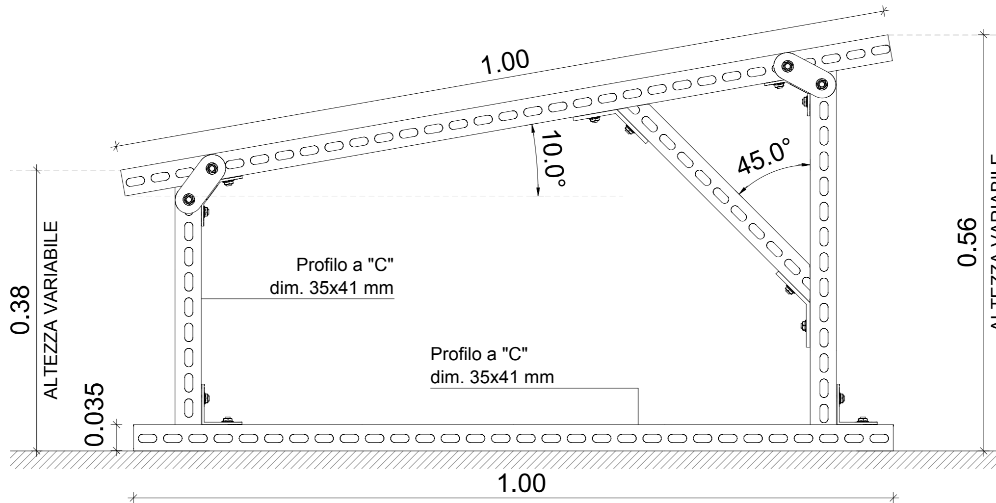
Prospetto - scala 1:5
